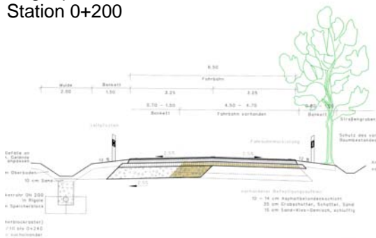
Regelquerschnitt bei Station 0+200
